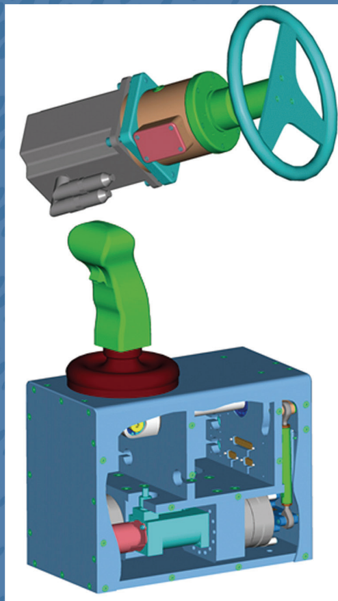
反力装置 (ステアリング、シフト、ペダルなど) ※特注品も承ります。
